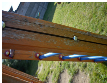
Rozszczepiona belka drabinki
