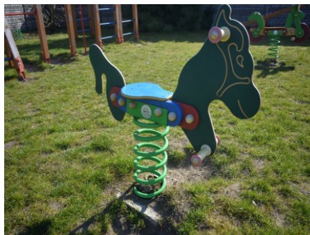
Odsłonięty, wystający fundament bujaka
