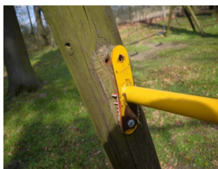
Uszkodzone mocowanie drążka
